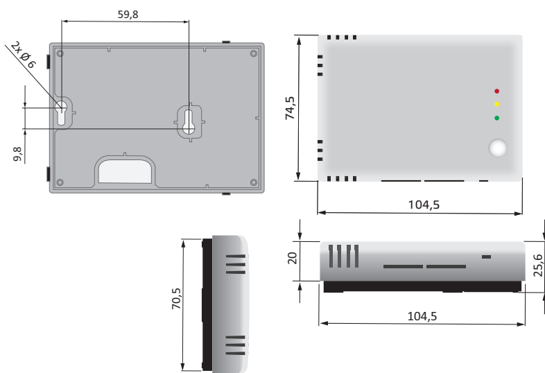
Фиг. 2 Монтажни размери
