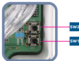
Фиг. 9 Бутони за стартиране на процедури за калибриране и възстановяване на фабричните Modbus настройки
