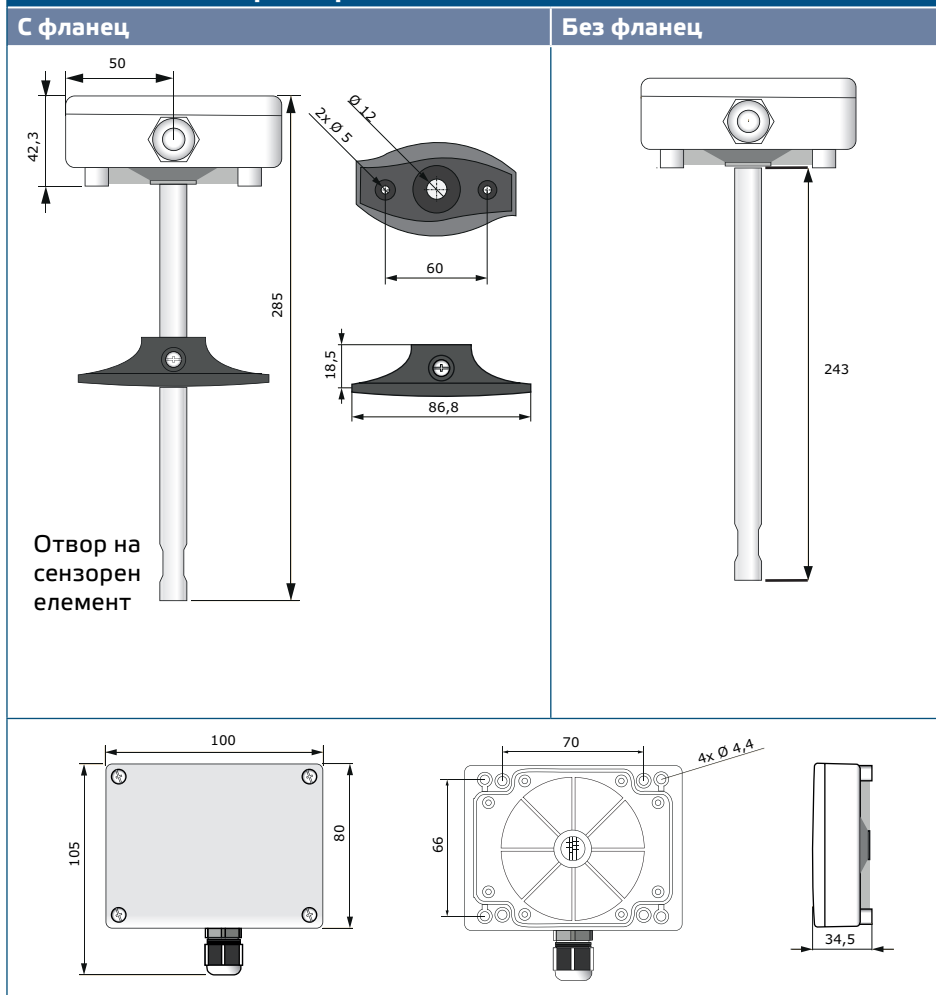
Фиг. 1 Монтажни размери
