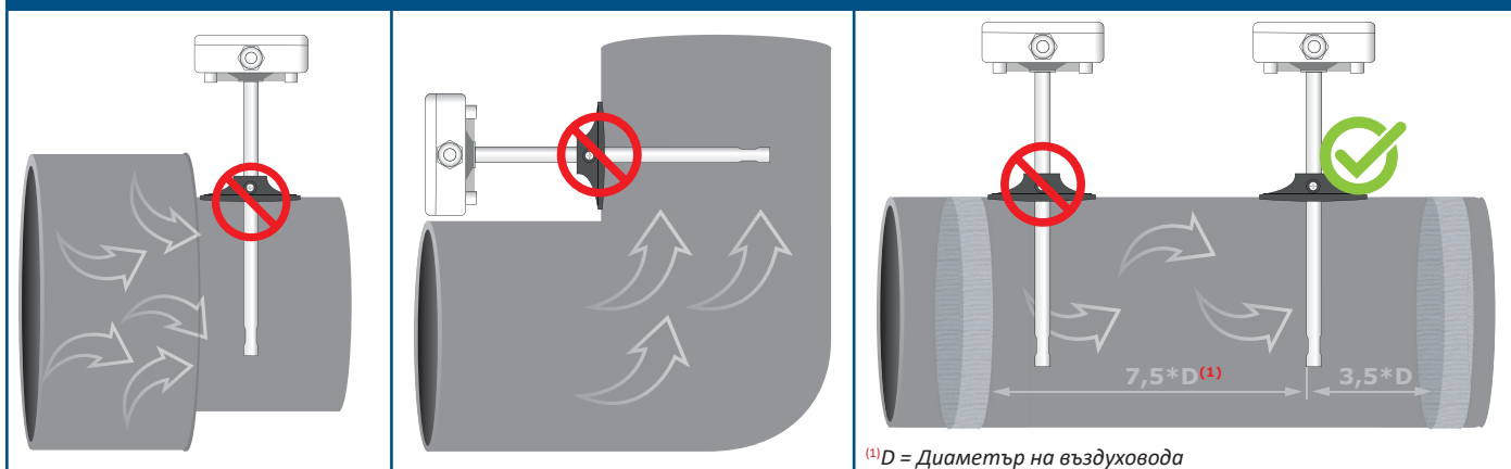
Фиг. 3 Изисквания за монтаж
