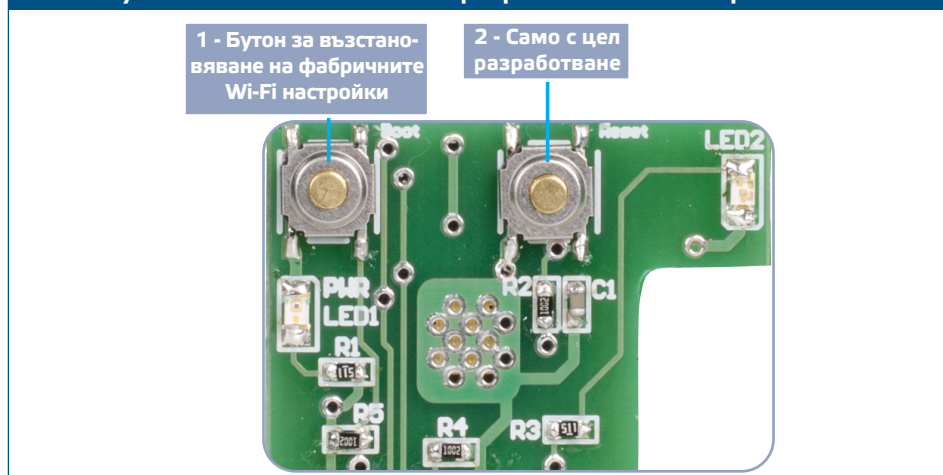
Фиг. 5 Бутон за възстановяване на фабричните Wi-Fi настройки
